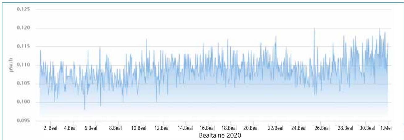
Fíor 11. Monatóireacht ar Ráta Dáileoige na Gámaradaíochta Comhthimpeallaí ar Eastát Chaisleán Bhaile Sheáin, Co. Loch Garman
